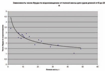
Рис. 8. Изменение числа Фруда (по водоизмещению) по интервалу изменения полной массы
