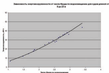
Рис. 11. Изменение энерговооруженности судов по интервалу числа Фруда по водоизмещению
