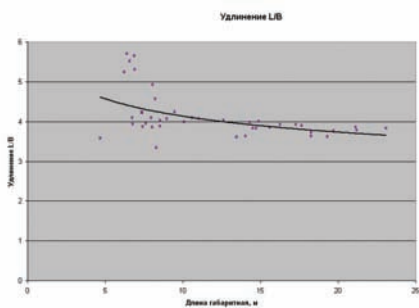
Рис. 9. Изменение отношения длины корпуса к ширине по интервалу изменения габаритной длины
